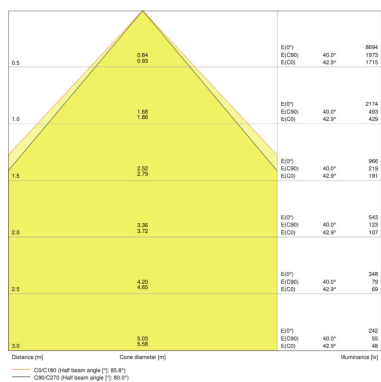
PL PFM 600 UGR19 36 W 4000 K
